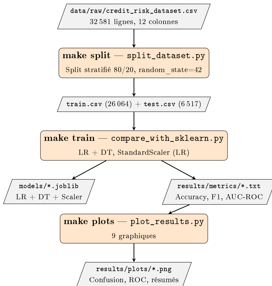
Figure 2.2: Flux du pipeline ML : $ make all exécute split → train → plots .
